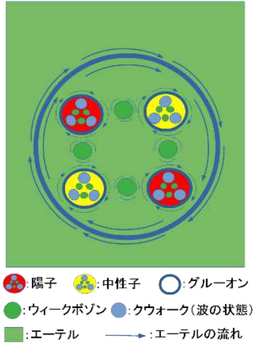
図2:α粒子
